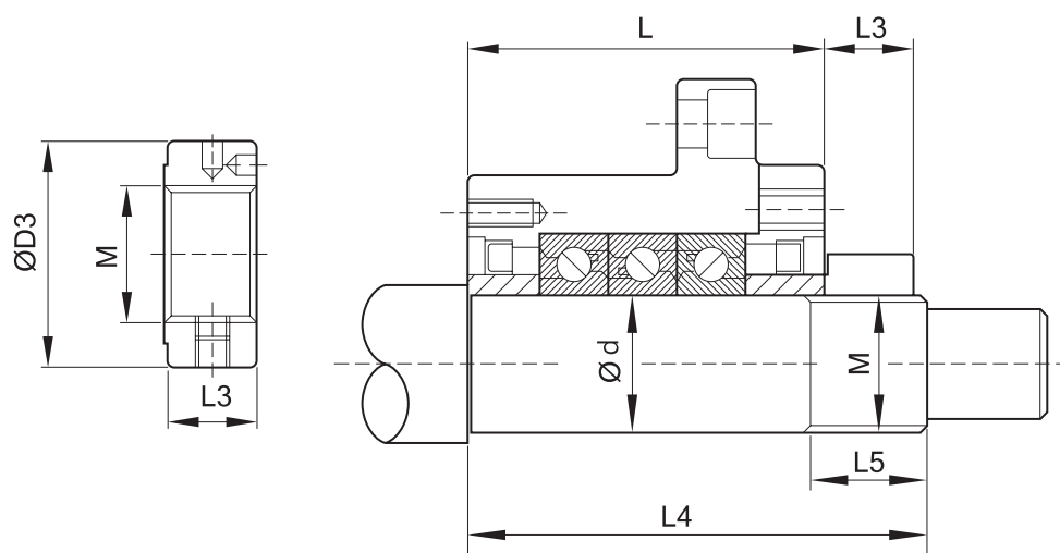
軸徑 Ød = 30 Shaft diameter
