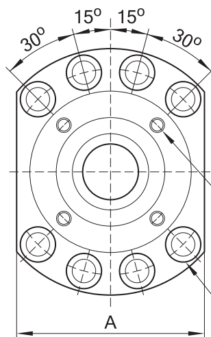
軸徑 Ød = 30 Shaft diameter
